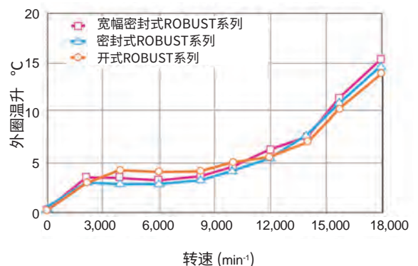
开式与密封式轴承温升对比
