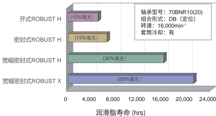
各系列产品润滑脂寿命对比
