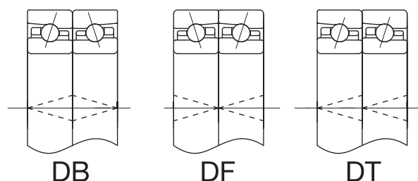
万能组合轴承的组合方式
